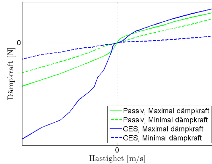
Figur 7.32: CES-dämparen
