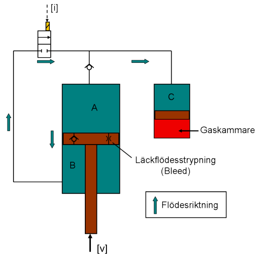
Figur 2.2. Skiss av oljeflödet vid kompressionslag.
