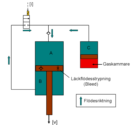
Figur 2.3. Skiss av oljeflödet vid returslag.
